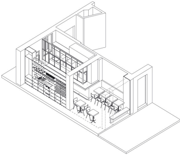
HOLIDAY CAFÉ_AXONOMÉTRIE
