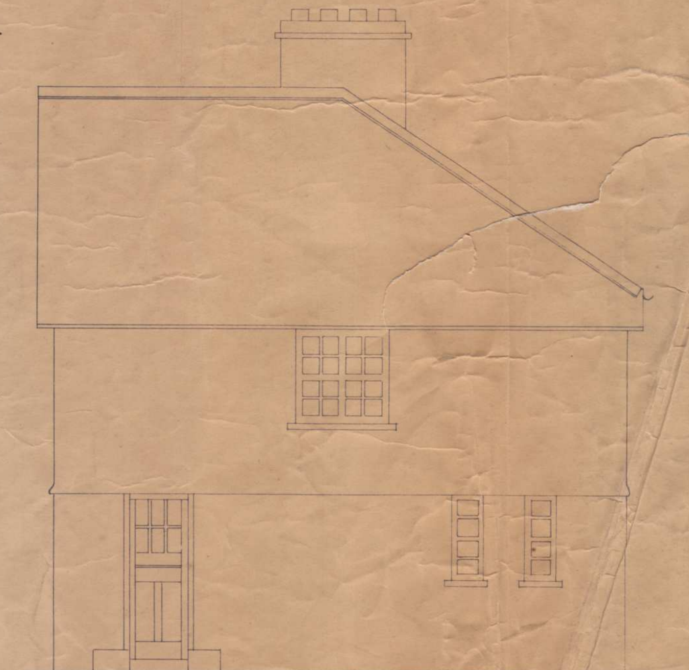
- END ELEVATION -
