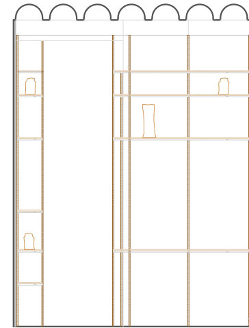
Sección Trans. 3-3'
