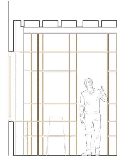
Sección Trans. 4-4'
