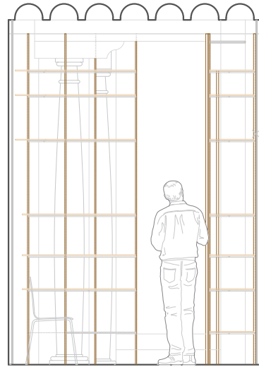
Sección Trans. 2-2'
