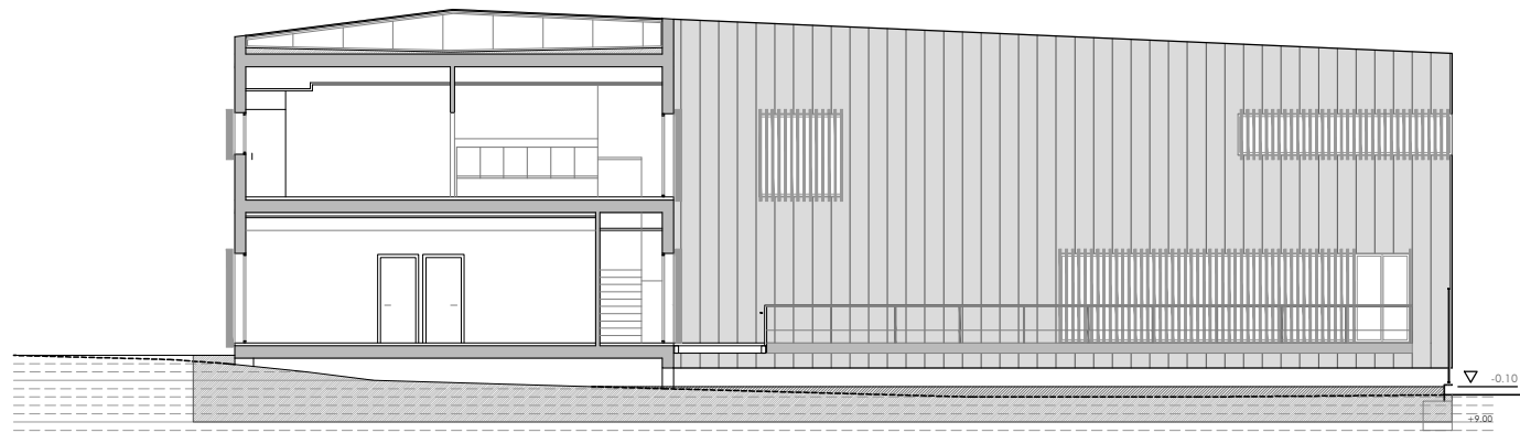
SECCIÓN C
