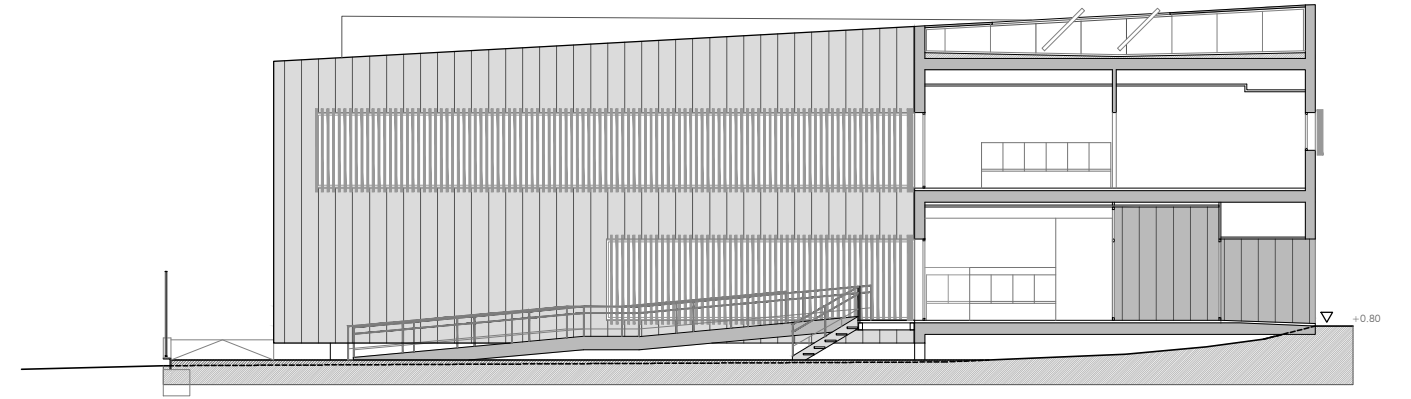
SECCIÓN B
