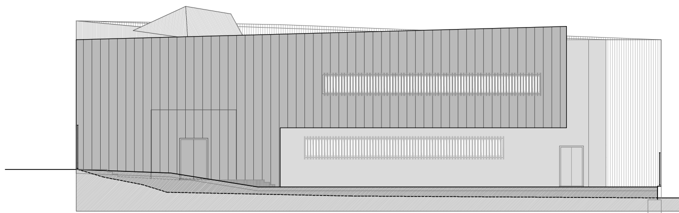
ALZADO SUR
