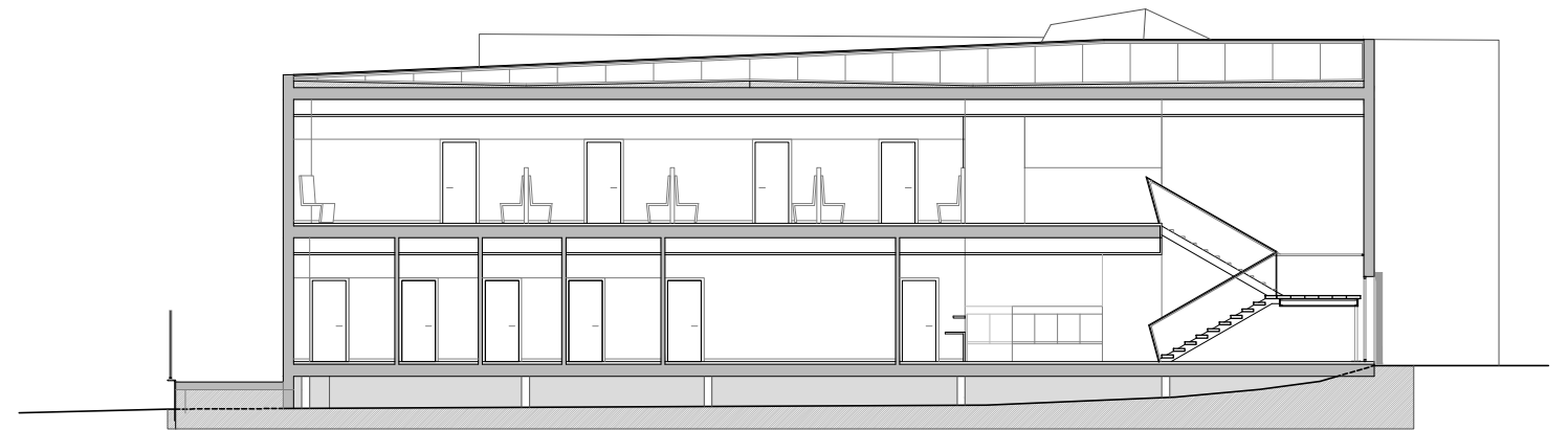
SECCIÓN E
