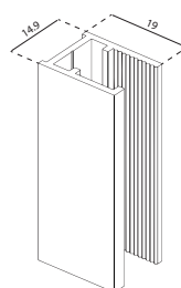
PERFIL FIJO U D-2162
