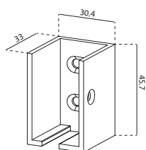
SOPORTE GUÍA D-2094
