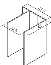
PERFIL EXPANSOR D-2055
