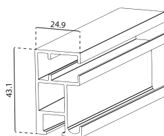
GUÍA SUPERIOR D-2094
