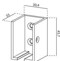
SOPORTE GUÍA D-2094
