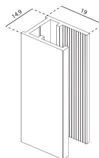
PERFIL FIJO D-2162
