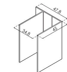
PERFIL EXPANSOR D-2055
