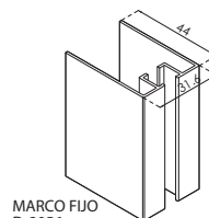
MARCO FIJO D-2056
