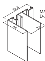
PERFIL EXPANSOR D-2055
