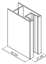
MARCO CABINA D-2029
