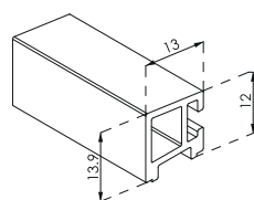
PERFIL BASE ALUMINIO D-2091
