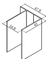
PERFIL EXPANSOR D-2055
