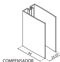
COMPENSADOR CABINA D-2018
