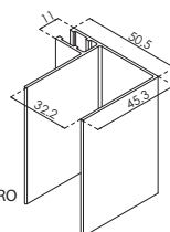
ESQUINERO D-2054
