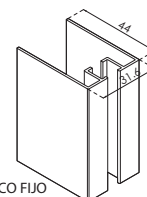
MARCO FIJO D-2056
