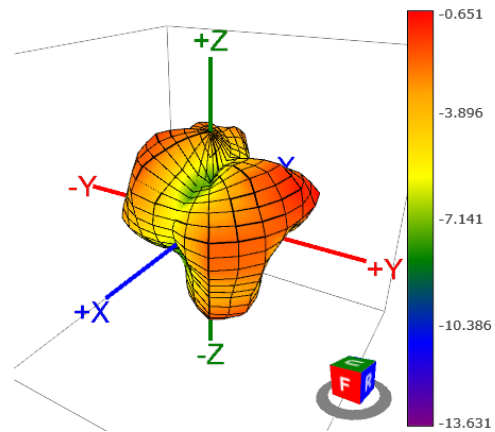
960MHz (dBi)
