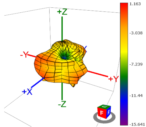
2690MHz (dBi)
