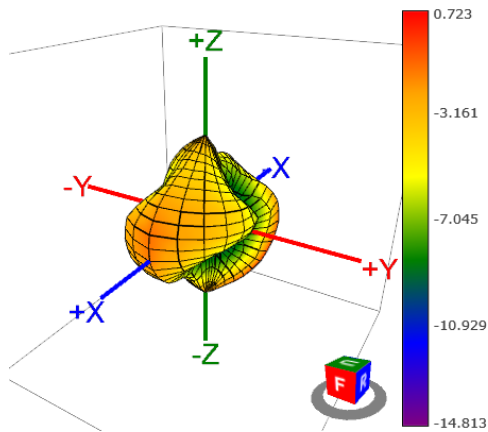
704MHz (dBi)
