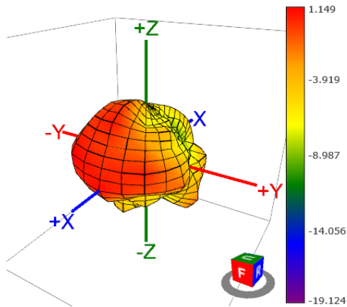
2300MHz (dBi)
