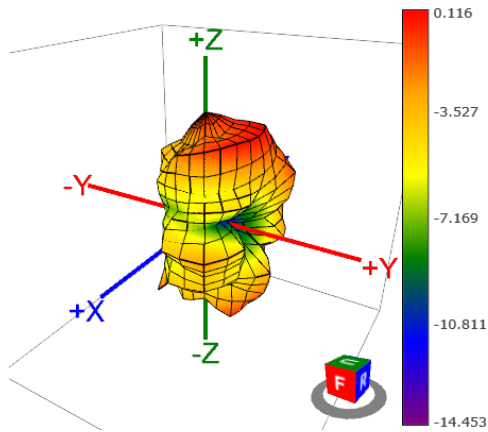
3300MHz (dBi)
