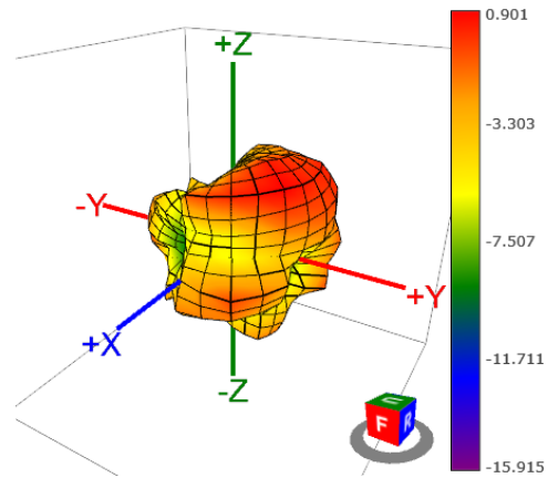
3800MHz (dBi)
