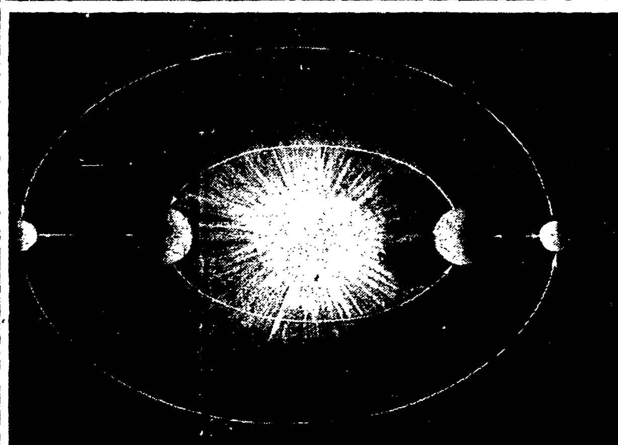
Nella loro corsa, Marte e la Terra si vengono a trovare sulla stessa linea col sole (in opposizione) ogni 773 giorni. Ma la distanza tra i due pianeti (posizione a destra) è minima solo ogni 15 anni; la data cadrà il 10 settembre prossimo
