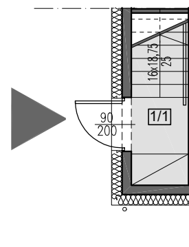
RZUT PARTERU
