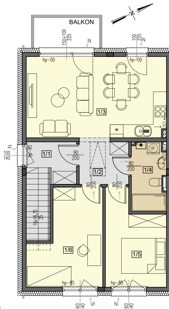
RZUT PODDASZA
