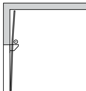
Prowadzenie VU z obniżonym wałem sprężyny skrętnej
