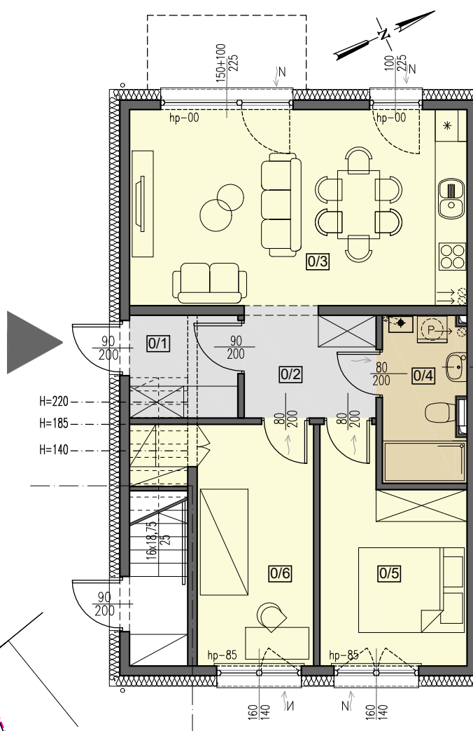
RZUT PARTERU
