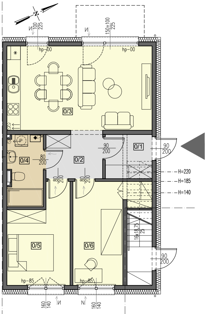
RZUT PARTERU
