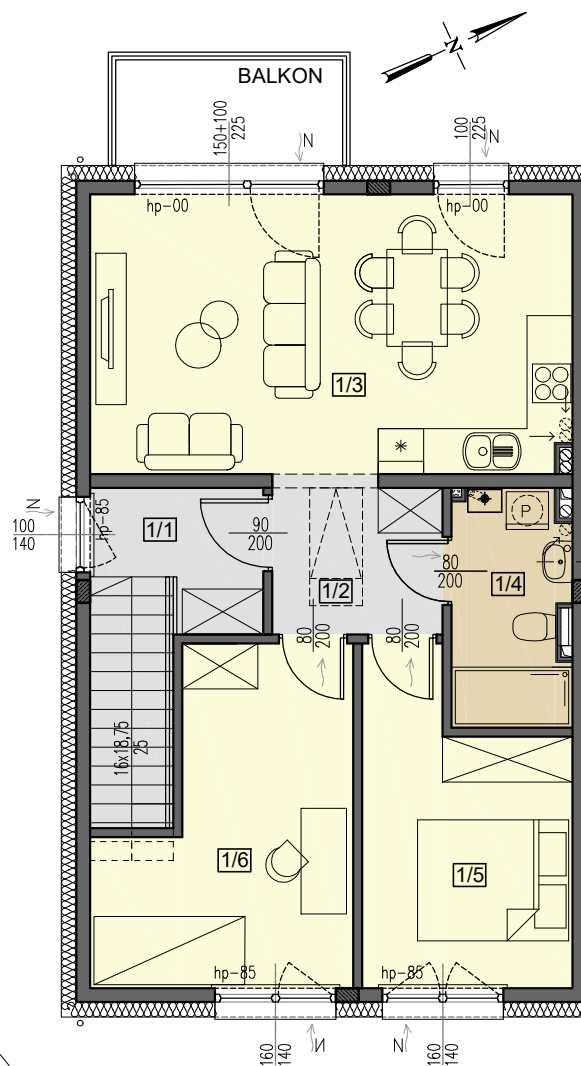
RZUT PODDASZA
