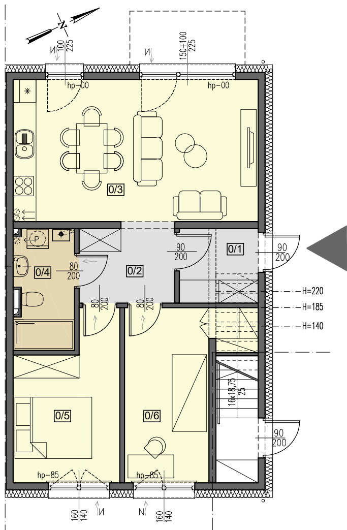
RZUT PARTERU
