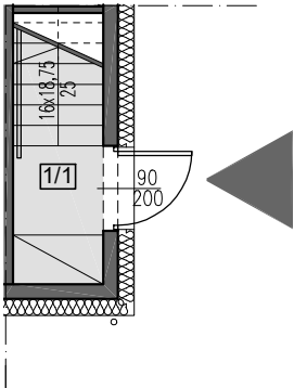
RZUT PARTERU
