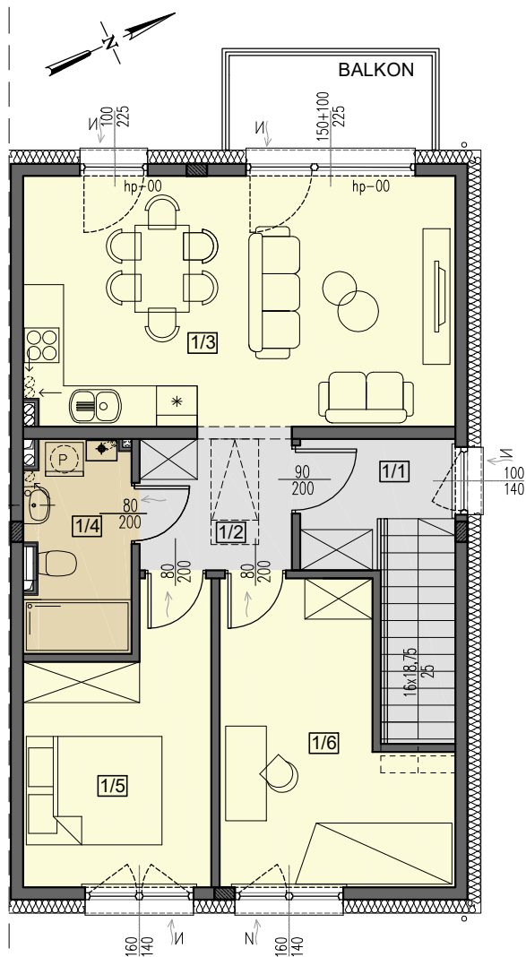
RZUT PODDASZA
