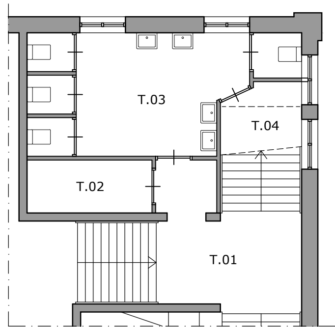
tussenvloer 1810+P
