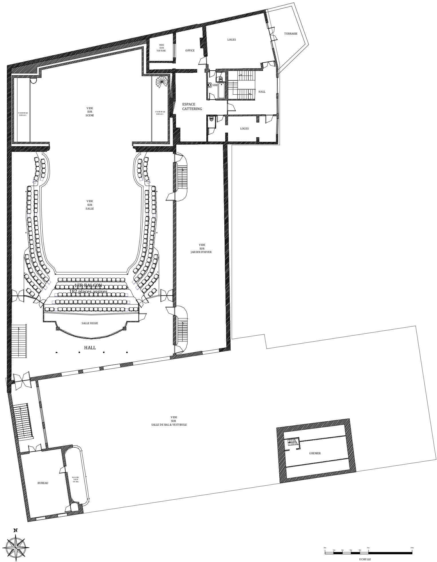
1er ETAGE
