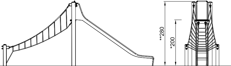
COR669101 1:100
