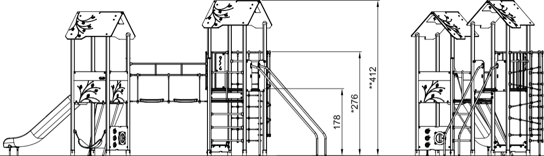
PCM211703-xx01 1:100
