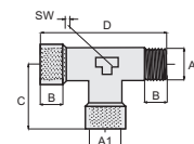
raccord taraudé/fileté
