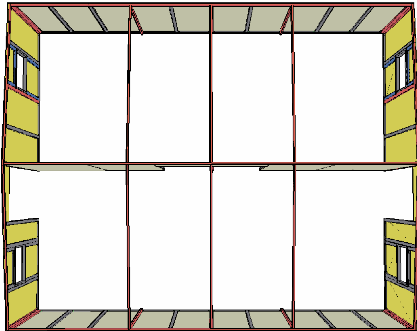
DISTRIBUCION EN PLANTA MEDIDAS 6.10 X 4.90 MTS
