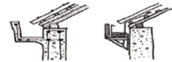
Calceira feita em betão
