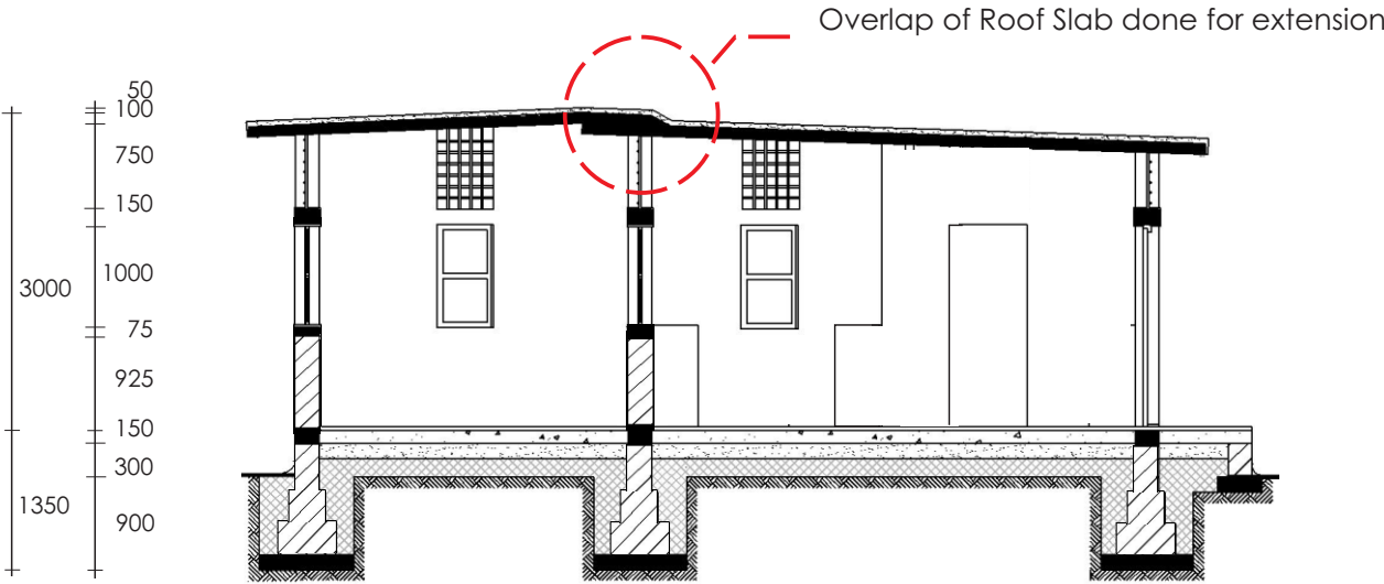
Section D-D
