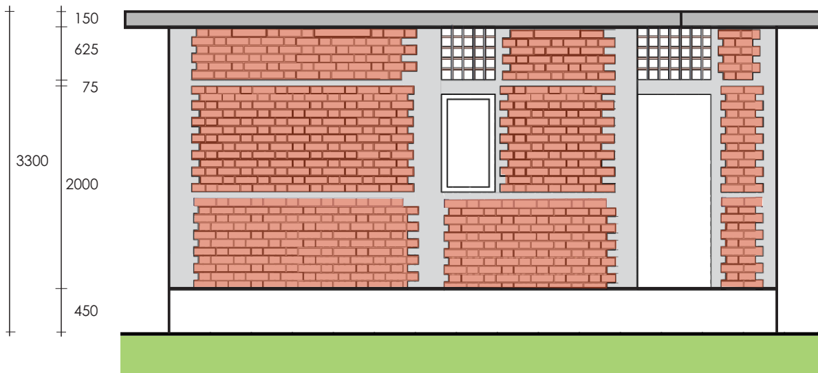
Right Elevation
