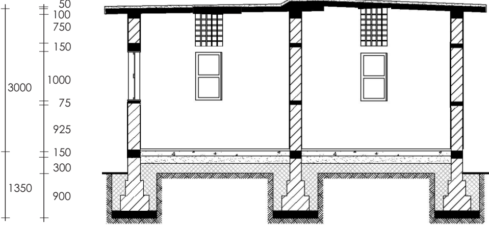
Section D-D
