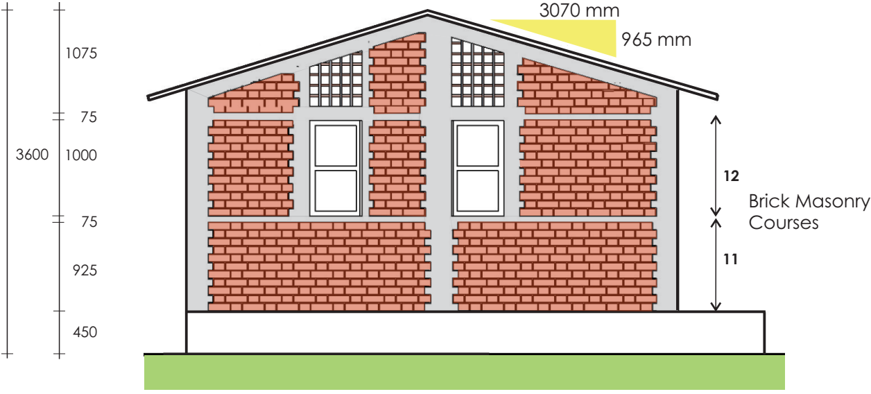
Right Elevation
