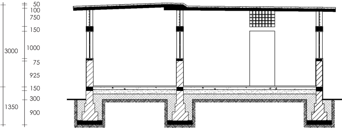
Section D-D
