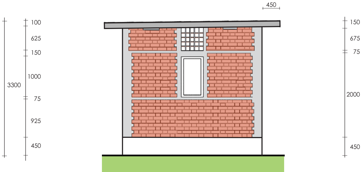
Right Elevation
