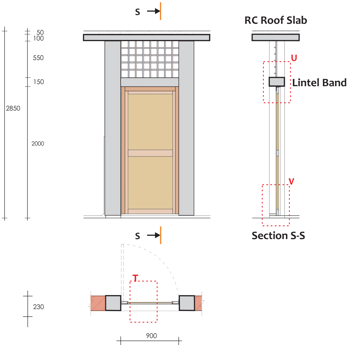
Door Details
