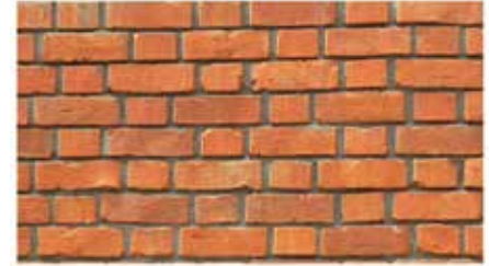
फ्लेमिस जोडाइ (Flemish Bond)
