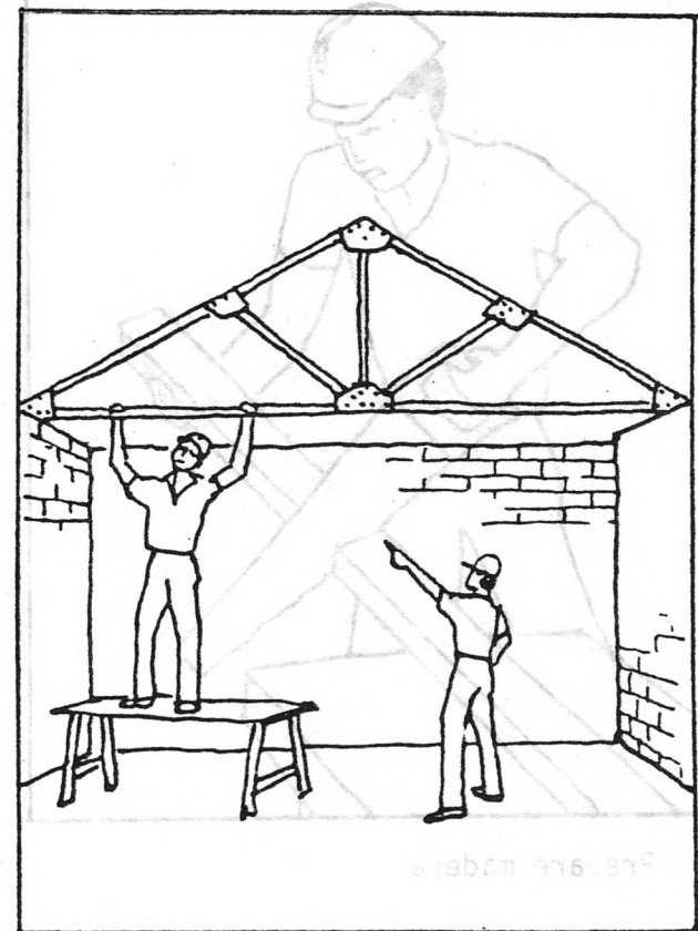
Coloque Cercha
