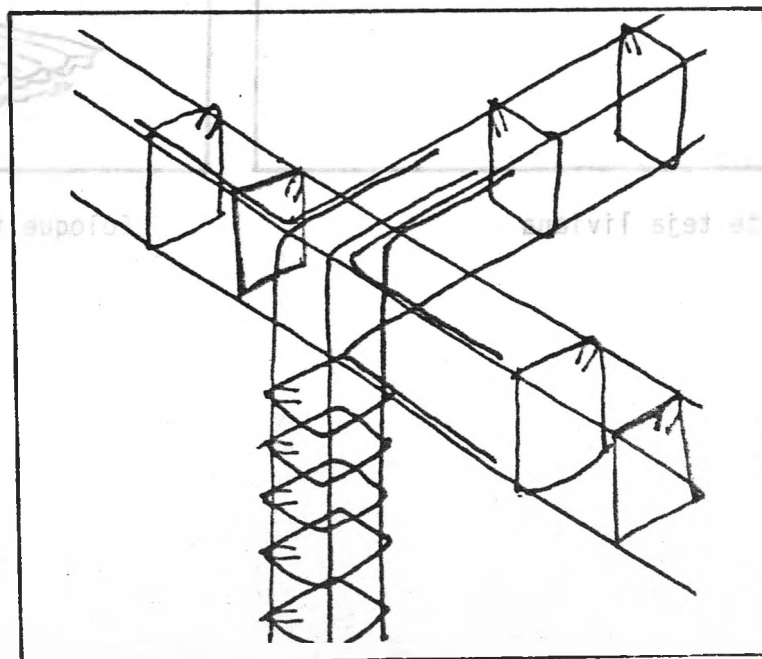
Unión de columneta con vigas de amarre en "T"
