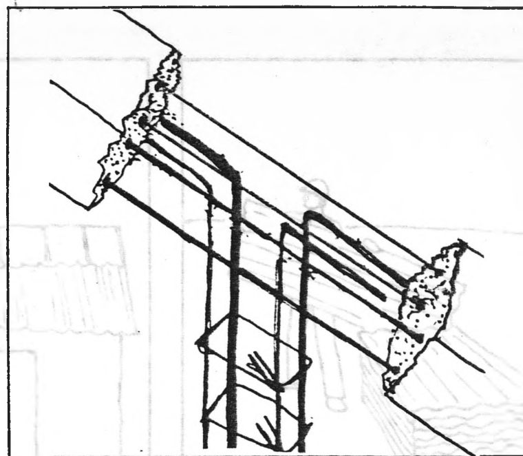
Anclaje de columneta nueva en viga existente
