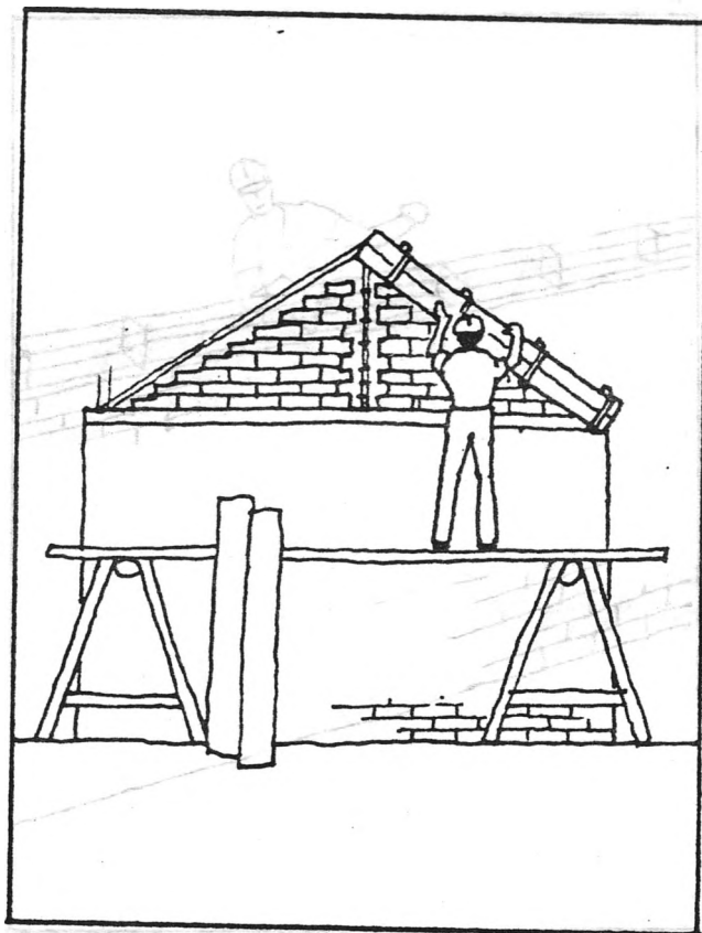
Formaletee (encofre) viga de corona y columneta
