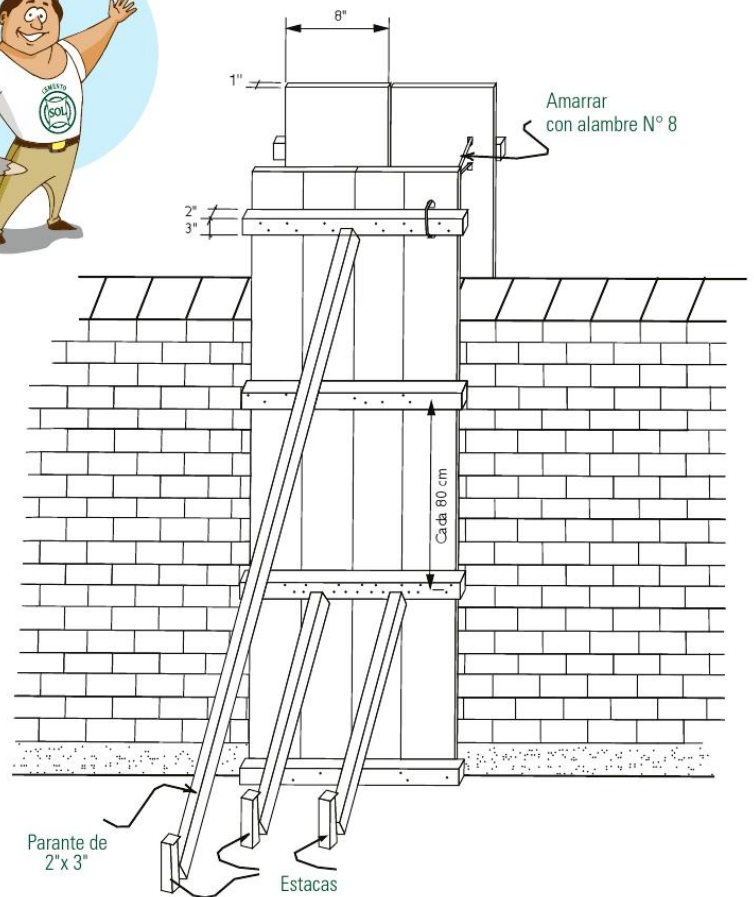
ENCOFRADO DE CARAS
