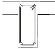
4 cm al estribo VIGAS
