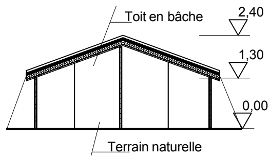
Façade Est
