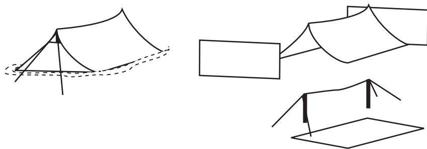
Diagrama explodido mostrando a cobertura, porta e chão separados. A porta e o chão foram cortadas da mesma lona de plástico.
