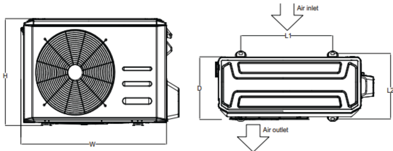
Fig. 3 — Dimensions
