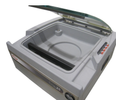
Kammare i livsmedelsgodkänd teknopolymer med inbyggd svetslist
