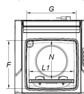
L1 260 • N 235 • G 300 • F 290 mm
