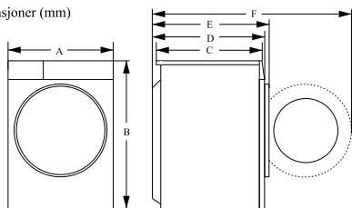
Dimensjoner (mm)
