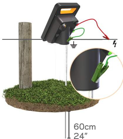
Puesta a tierra para el Paso 3 (d.)
