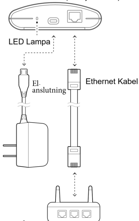
GATEWAY ULTRA Enhet (visas från sidan)
