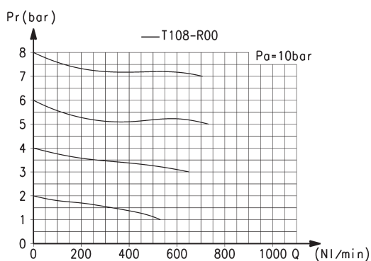
Diagramma di portata per modello: T108-R00
