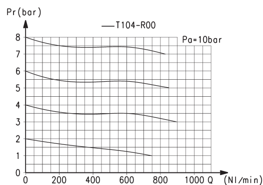
Diagramma di portata per modello: T104-R00
